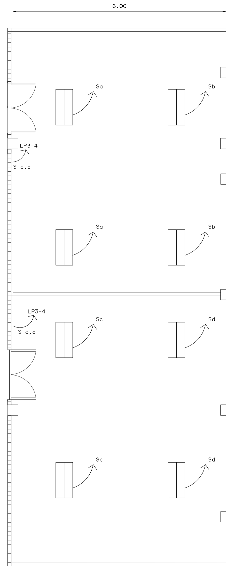
แปลนปรับปรุงห้องซ่อมดนตรี ระบบไฟฟ้า (แสงสว่าง)
