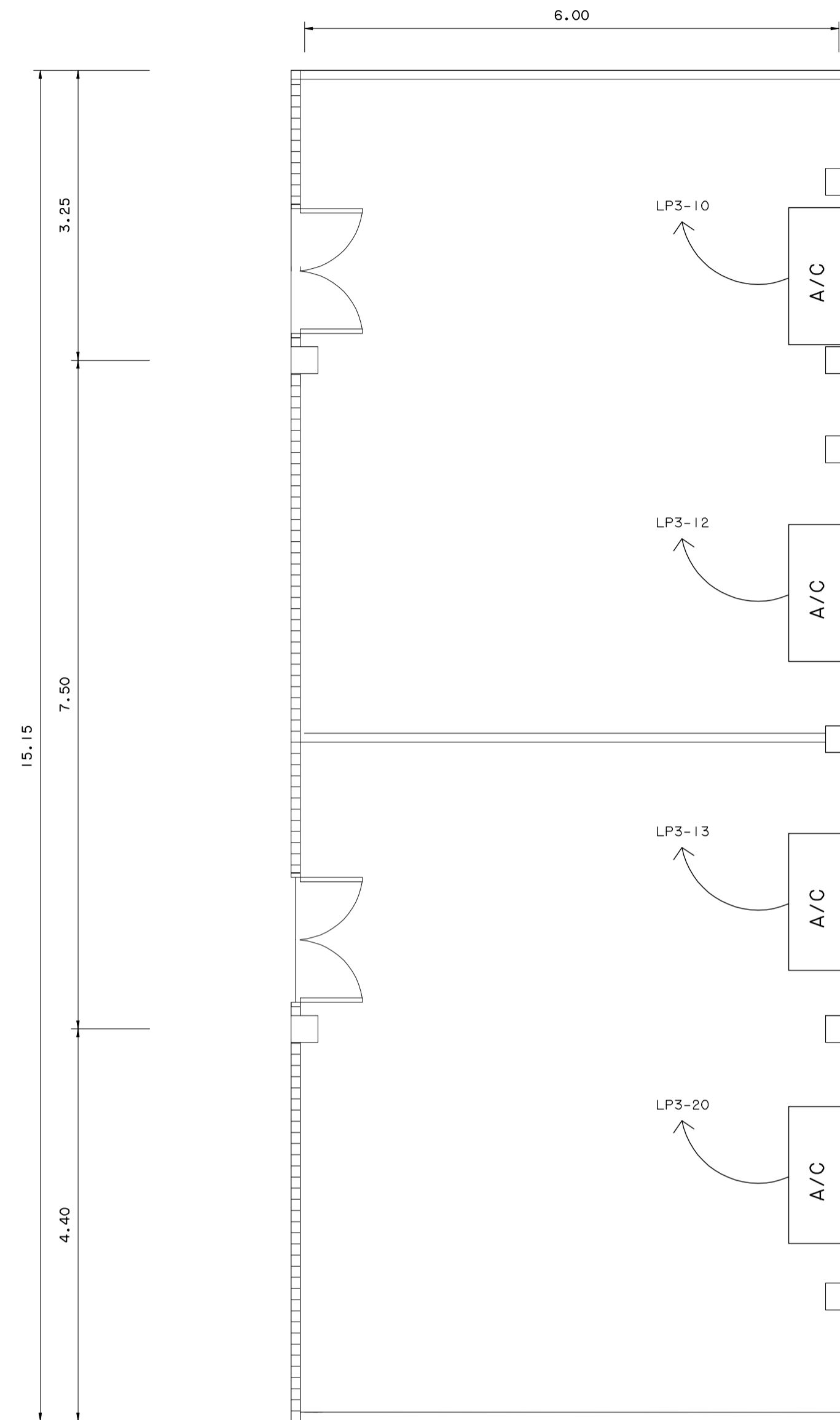
แผนปรับปรุงห้องห้องซัอมดนตรี ระบบปรับอากาศ มาตราส่วน 1 : 50
