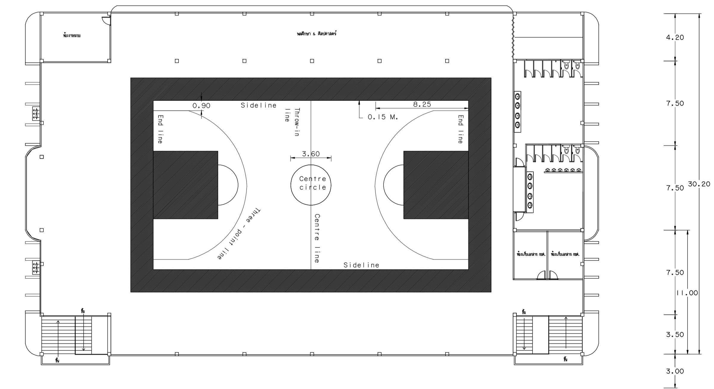
สัญลักษณ์ และรายการ งานตีเส้น และสีพื้นสนามบาส แปลนพื้นชั้น 2 งานตีเส้น และสีพื้นสนามบาส มาตราส่วน 1 : 200
