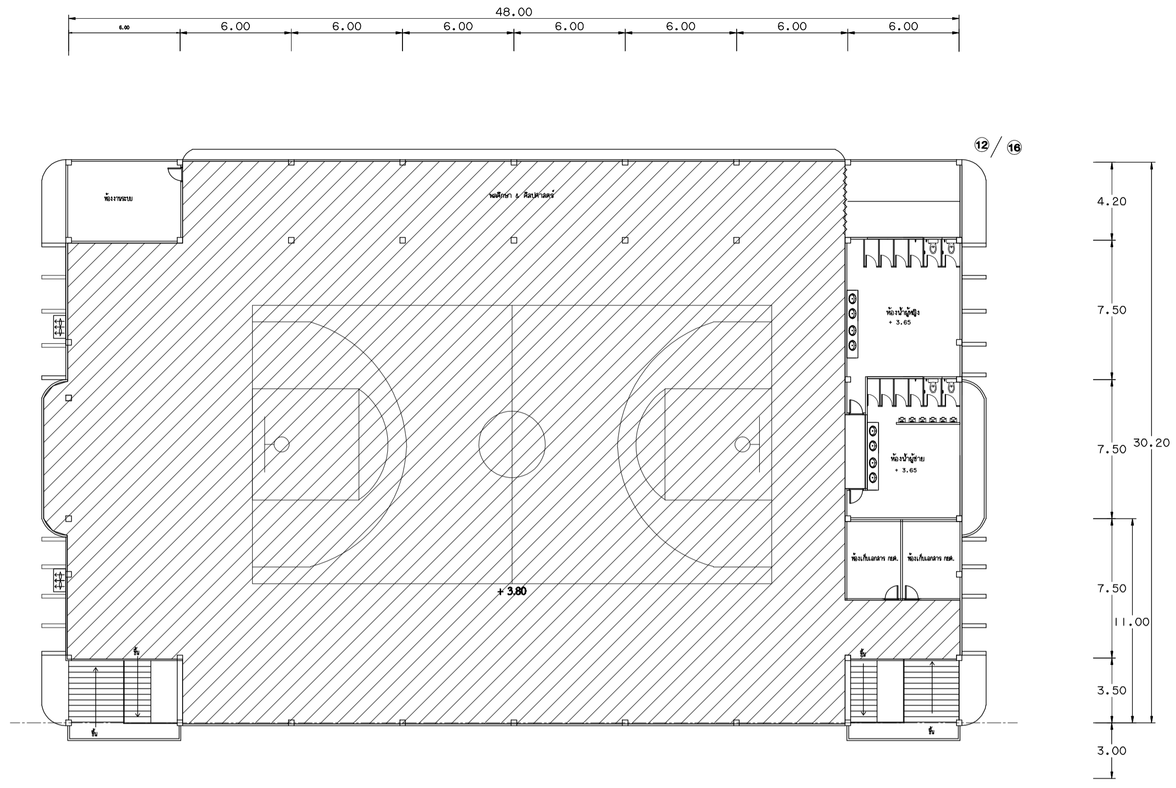
สัญลักษณ์ และรายการ งานขีดพื้น-ย้อมสีธรรมชาติ แปลนพื้นชั้น 2 งานขีดพื้น-ย้อมสีธรรมชาติ มาตราส่วน 1 : 200
