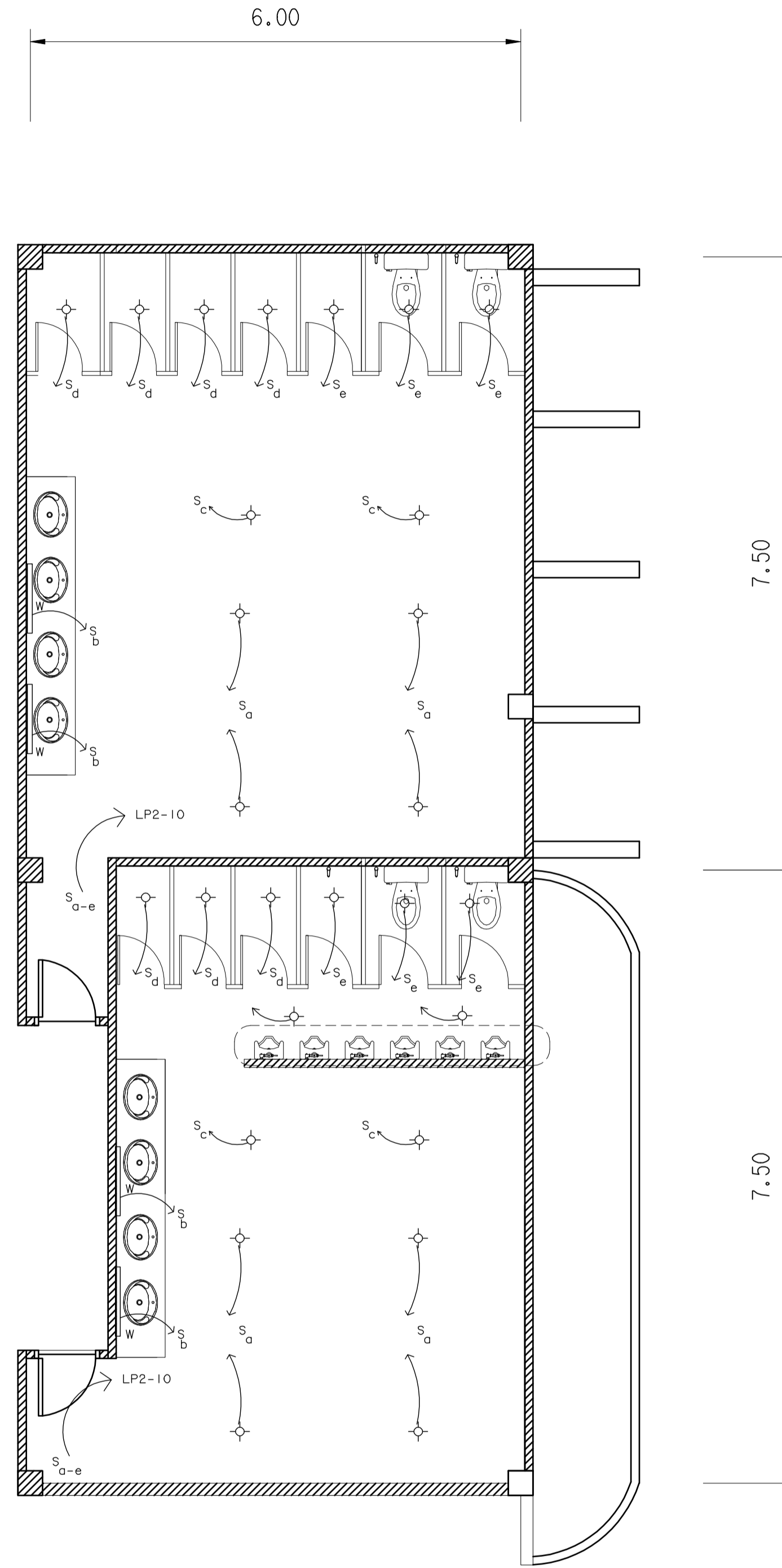
แปลนห้องน้ำชาย - ห้องน้ำหญิง ระบบไฟฟ้า(แสงสว่าง) มาตราส่วน 1 : 50
