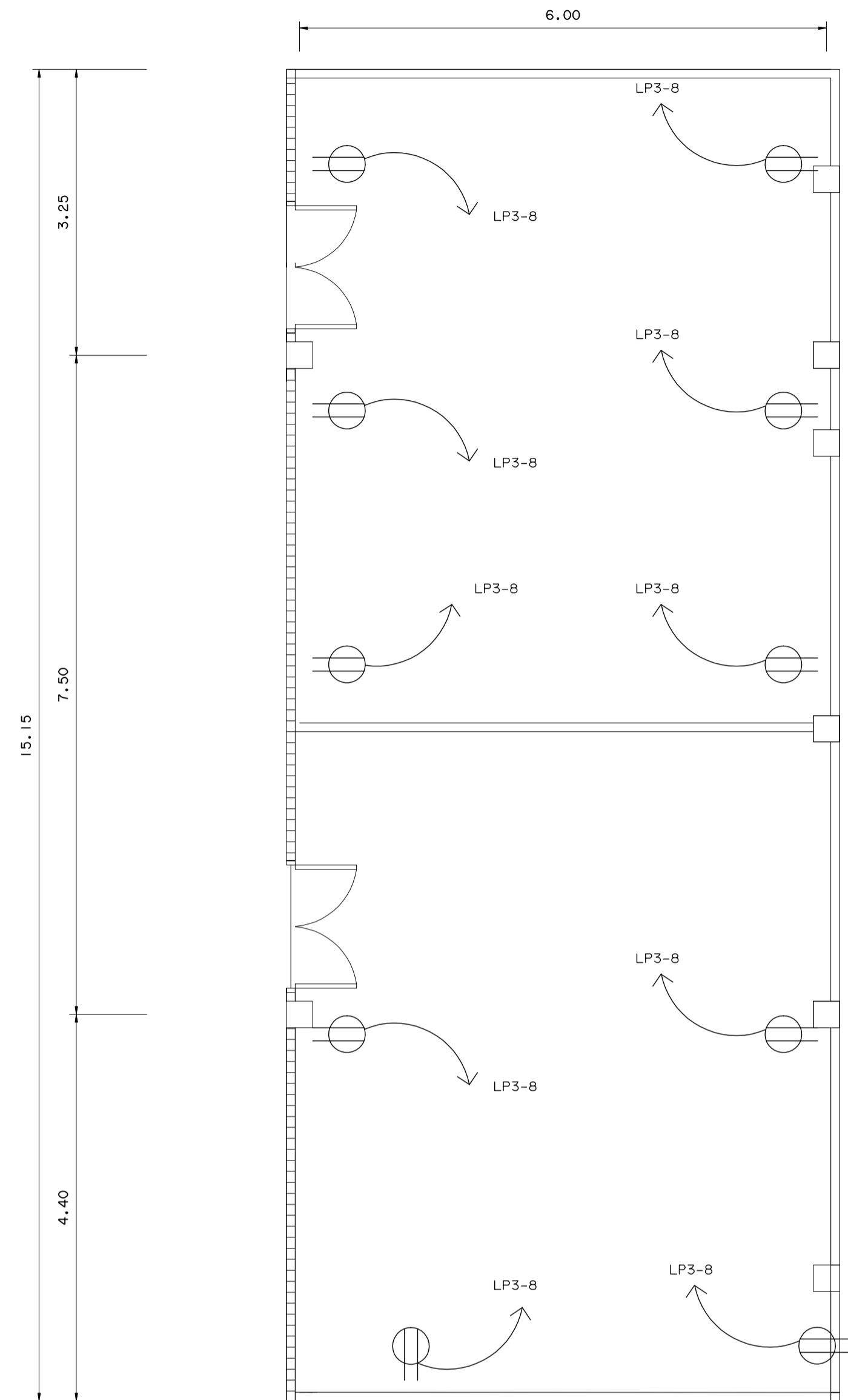
แปลนปรับปรุงห้องซ่อมดนตรี ระบบไฟฟ้า (ตัวรับ)
